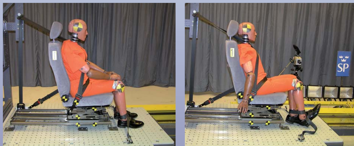
Crashtest-Fotos der Autoadapt 6-Wege-Basis im SP (schwedisches Test- und Forschungsinstitut). Die Fotosequenz zeigt die Situation vor und nach dem Test.
