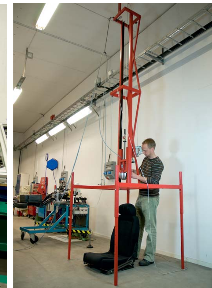
Vorbereitung eines Aufprallenergie tests an einem Sitz.
